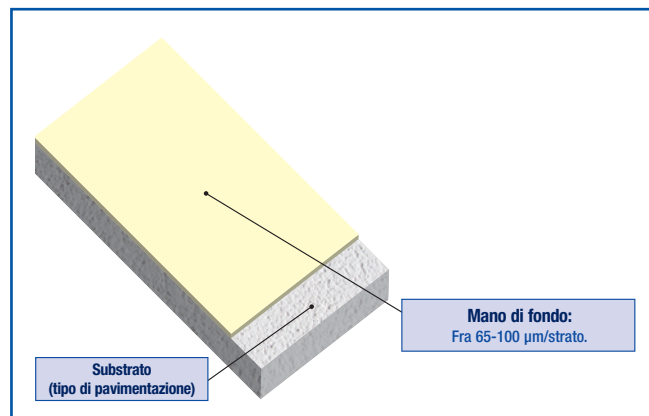
Sistema antipolvere
